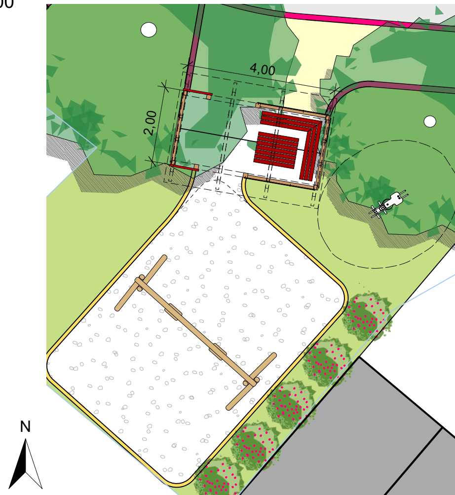
Planausschnitt mit Grundriss Pavillon M1:100
